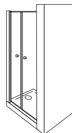
parete doccia con apertura 180° interno & esterno per installazione in nicchia / solution for niche with saloon door /
