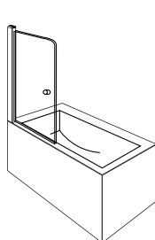
parete per vasca da bagno con apertura a 90° sia all'interno che all'esterno / foldable bath screen one part /
